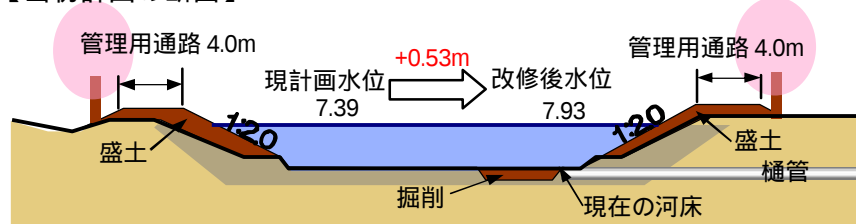
【当初計画の断面】
