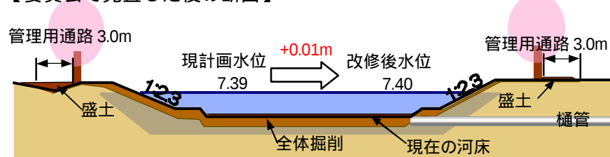
【委員会で見直した後の断面】
